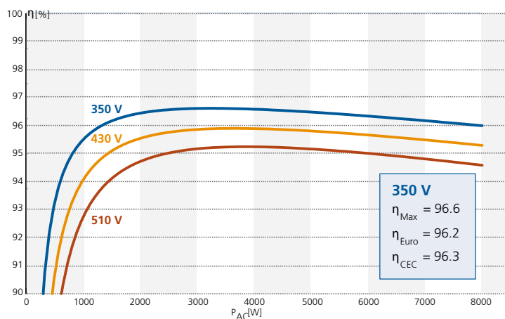
Wirkungsgradkennlinien Powador 9600
